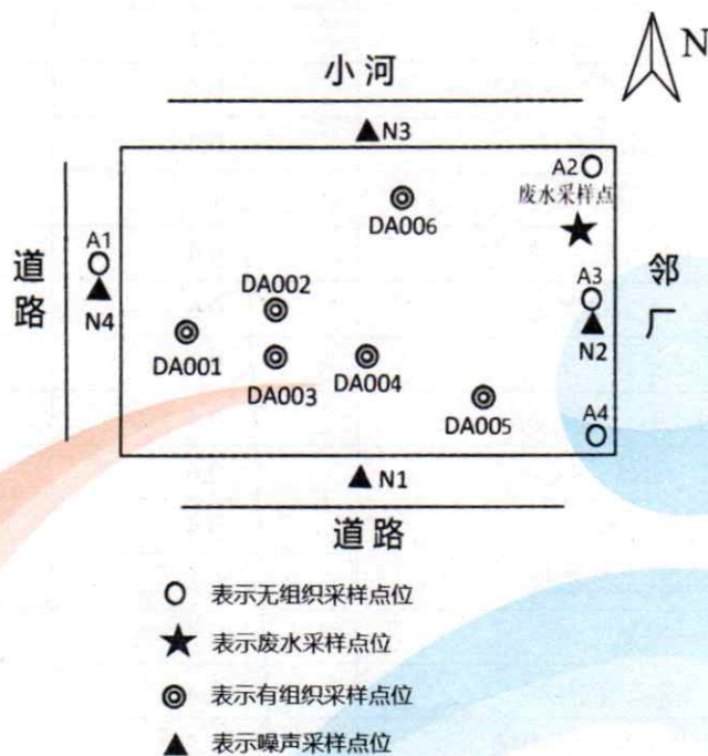
附图: 检测布点平面示意图
